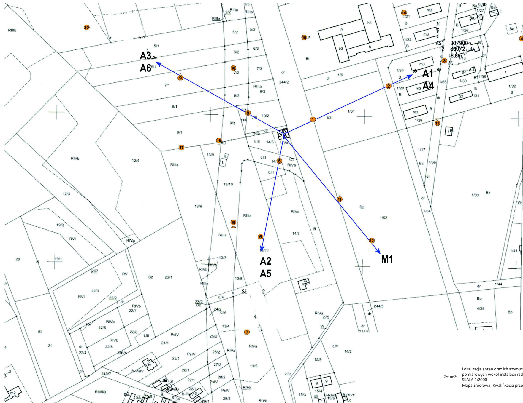
Azymuty anten T-Mobile
